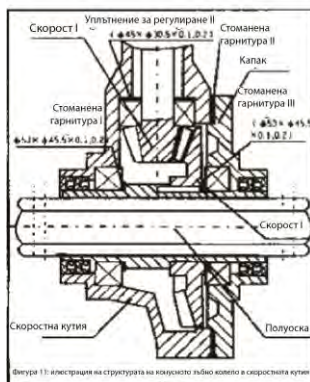
Фигура 11: илюстрация на структурата на колелото зъбно колело в скоростната кутия
