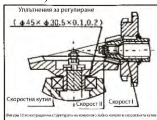
Фигура 10: илюстрация на структурата на колелото зъбно колело в скоростната кутия
